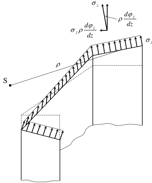
Sl. 2.6. Wagnerov efekt
