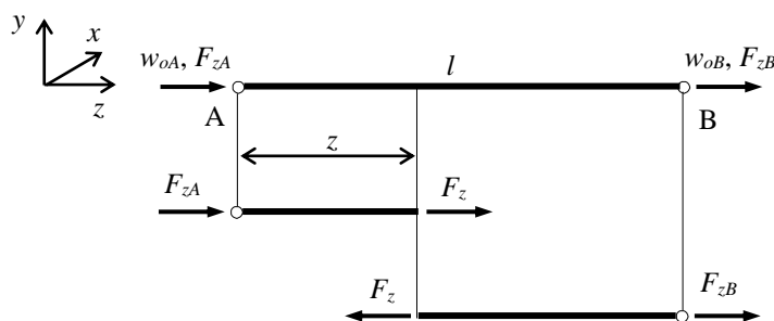
Sl. 3.3. Aksijalno opterećenje konačnog elementa: komponente pomaka i komponente sile
