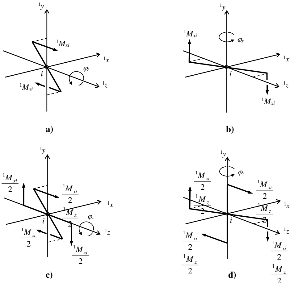
Sl. 3.20. Inkrementalne rotacije momenta {}^1M_{xi} oko koordinatnih osi: a) rotacija momenta {}^1M_{xi} -QT1 oko osi {}^1z ; b) rotacija momenta {}^1M_{xi} -QT2 oko osi {}^1y ; c) rotacija momenta {}^1M_{xi} -ST oko osi {}^1z ; d) rotacija momenta {}^1M_{xi} -ST oko osi {}^1y
